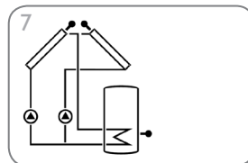
Système de chauffage solaire avec 2 capteurs et 1 réservoir (page 32)
