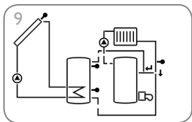
Système de chauffage solaire avec augmentation de la température de retour (page 41)
