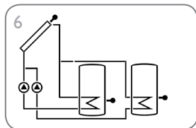
Système de chauffage solaire à 2 réservoirs avec logique de pompe (page 29)
