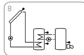
Système de chauffage solaire avec chauffage d'appoint à travers chaudière combustible solide (page 35)
