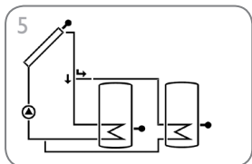
Système de chauffage solaire à 2 réservoirs avec logique de vanne (page 26)
