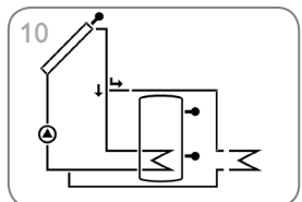
Système de chauffage solaire standard avec évacuation de l'excès de chaleur (page 44)
