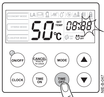
Fig.21 Bevestiging
