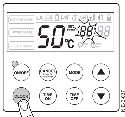
Fig.11 Afstelling
