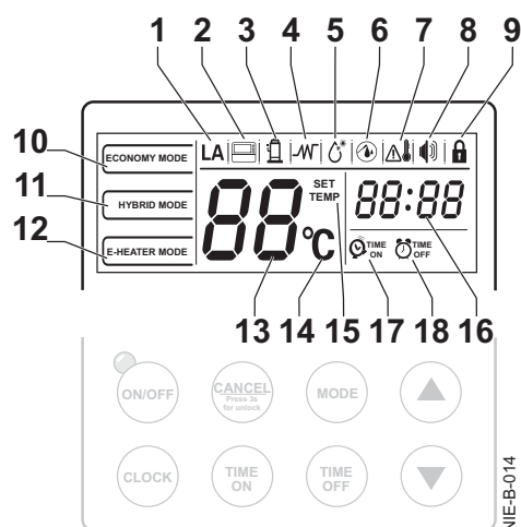
Fig.5 Displa
