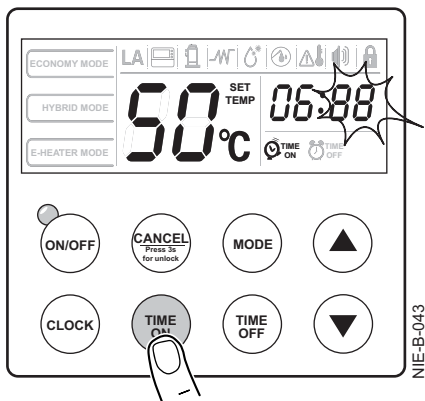
Abb.17 Bestätigung
