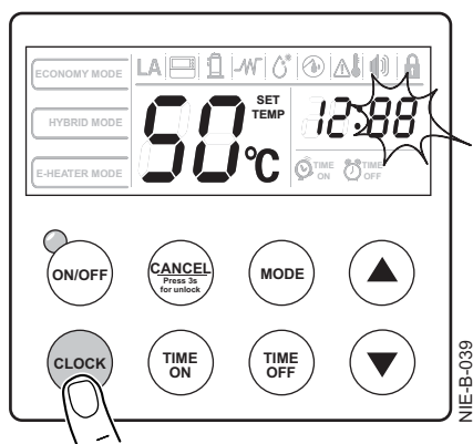
Abb.13 Bestätigung
