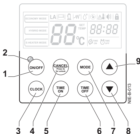
Abb.4 Die Bedientasten
