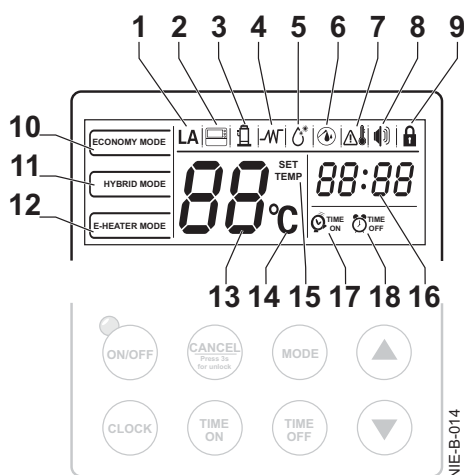
Abb.5 Das Display
