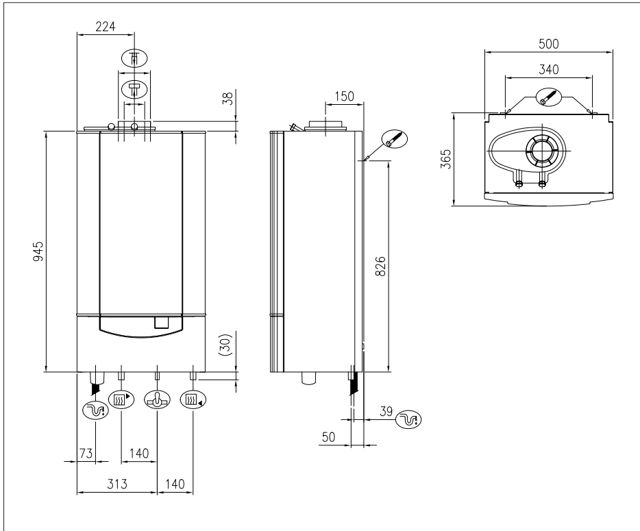
Afb. 04 Afmetingen Remeha Quinta 25s en 30s 03.W3H.79.00004
