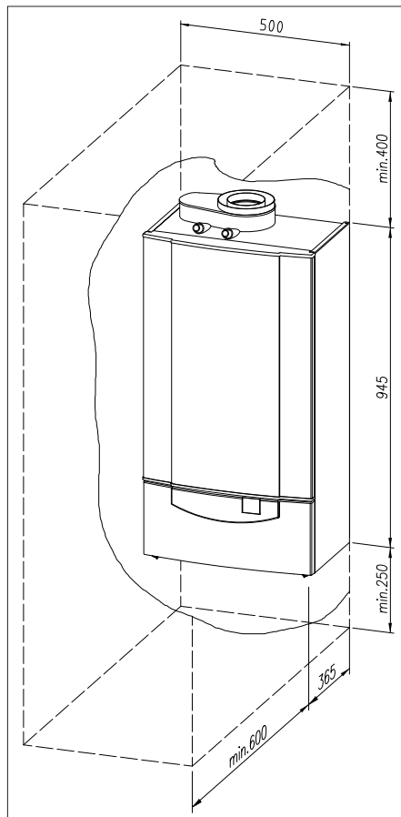
Afb. 07 Opstellingsruimte Remeha Quinta
