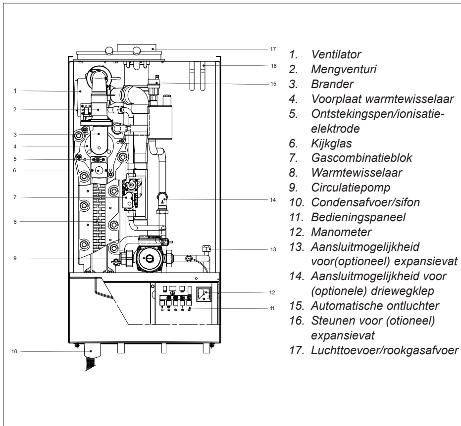
Afb. 02 Toesteluitvoering Quinta 25s en 30s (solotoestel)
