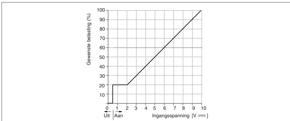
Afb. 22 Relatie tussen ingangsspanning en nominale belasting
