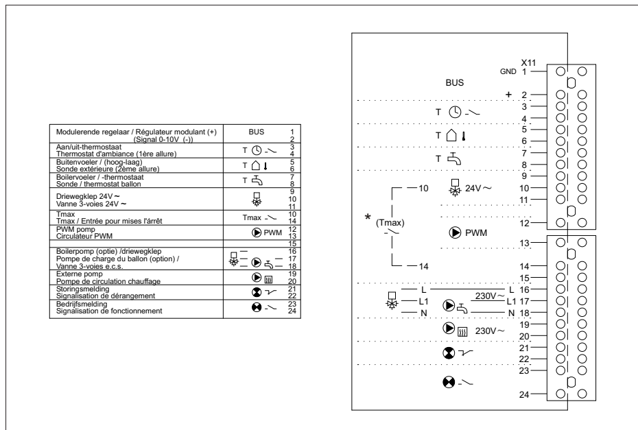
Afb. 18 Klemmenstrook
