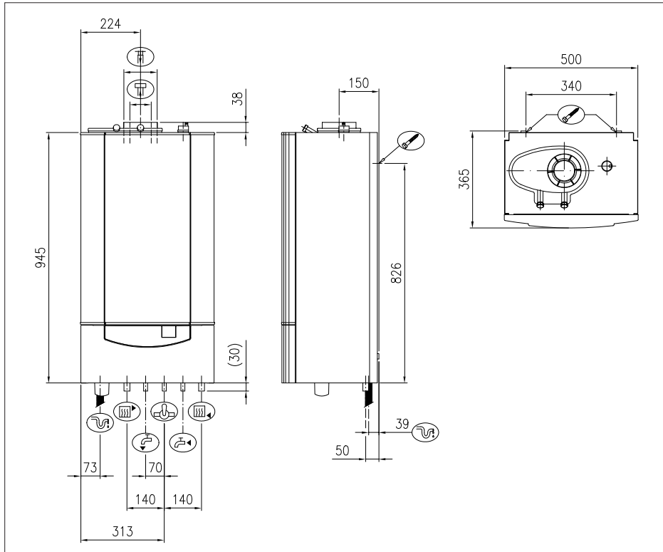
Afb. 03 Afmetingen Remeha Quinta 28c en 35c 03.W3H.79.00005
