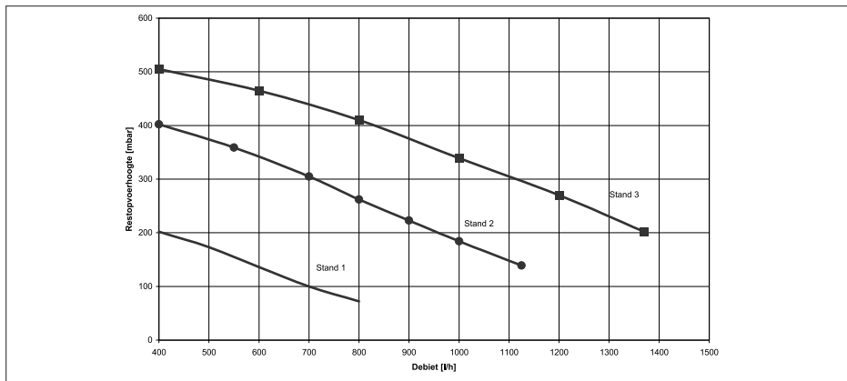
Afb. 15 Grafiek restopvoerhoogte Quinta 30s, 28c en 35c t.b.v. de c.v.-installatie
