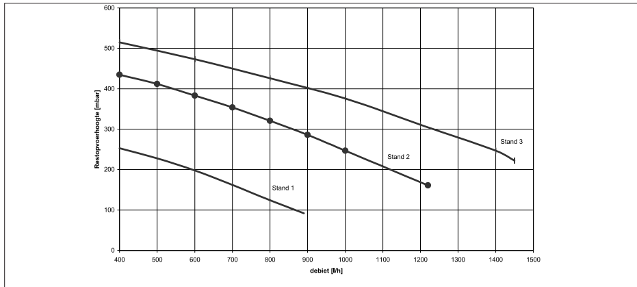
Afb. 14 Grafiek restopvoerhoogte Quinta 25s t.b.v. de c.v.-installatie
