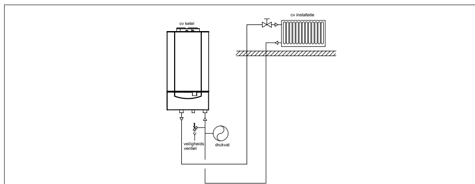
Afb. 13 Veiligheidsvoorzieningen bij Quinta 28c en Quinta 35c (bij Quinta 25s en Quinta 30s, veiligheidsventiel in de aanvoerleiding)
