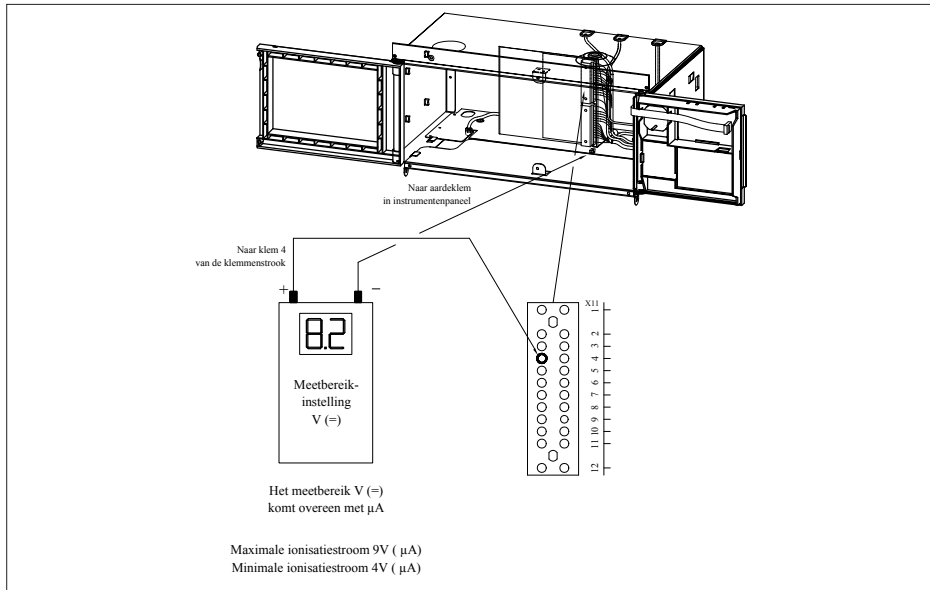
Afb. 26 Ionisatiemeting 00.V3H.79.00051
