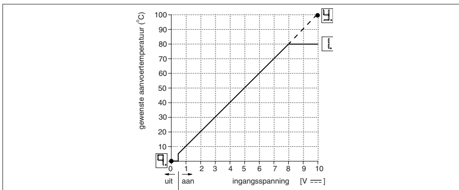
Afb. 21 Relatie tussen ingangsspanning en ketelaanvoertemperatuur
