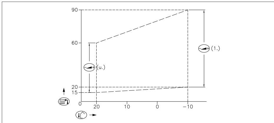
Afb. 23 Interne stooklijn
