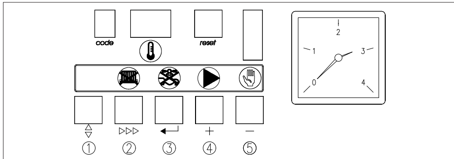
Afb. 05 Bedieningspaneel 00.W4H.79.00044
