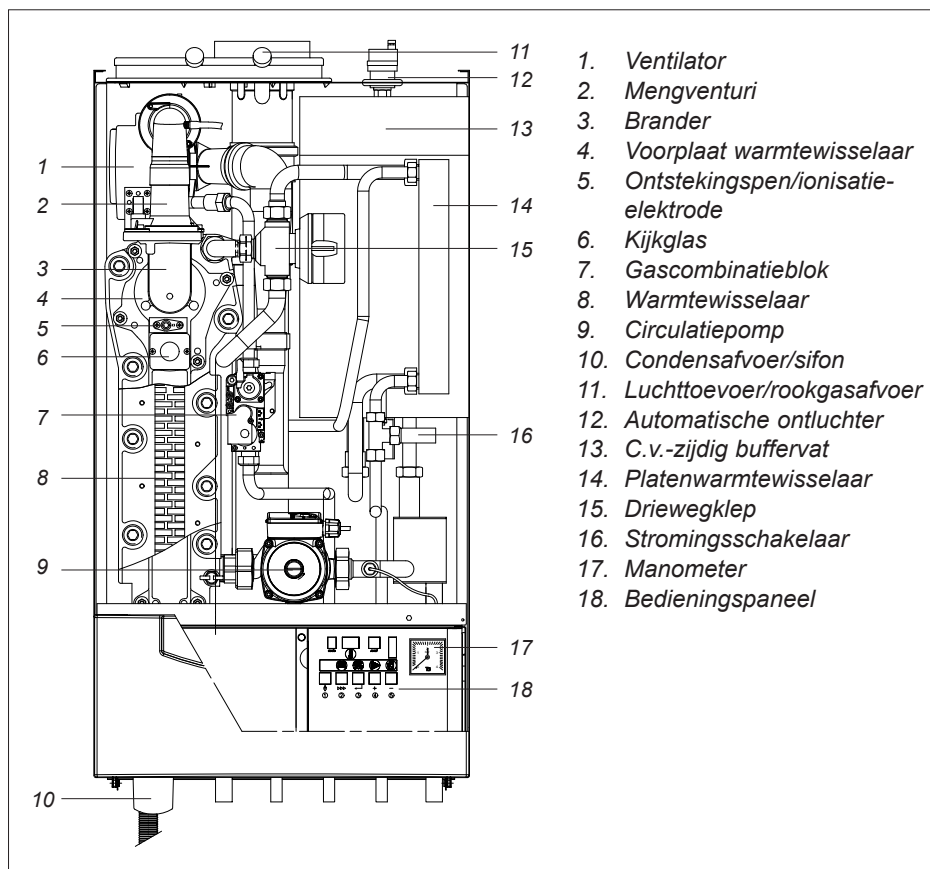
Afb. 01 Toesteluitvoering Quinta 28c en 35c (combtoestel met driewegklep en buffervat)
