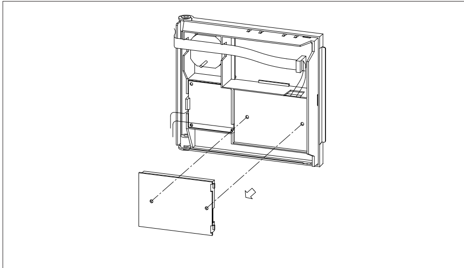
Afb. 20 Interface inbouw
