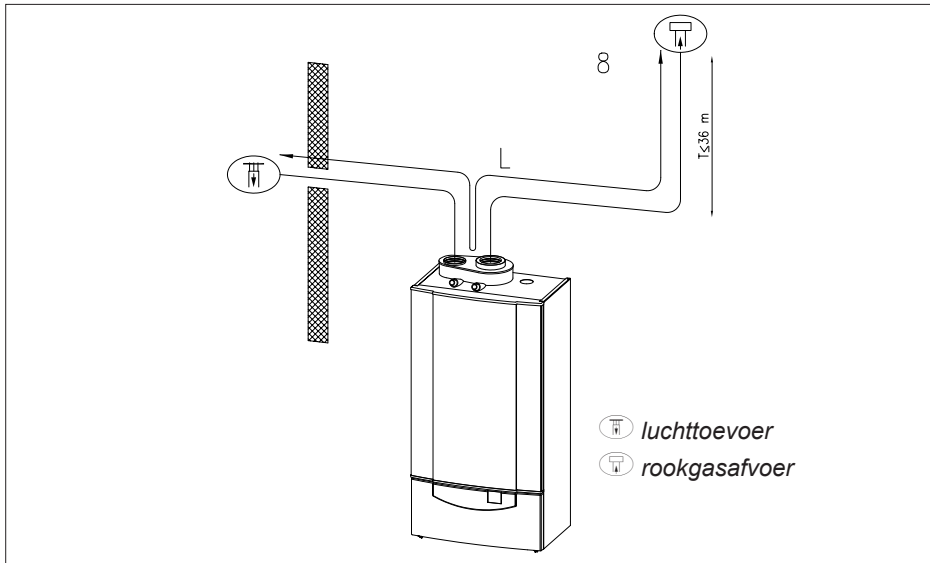
Afb. 12 Uitmondig in verschillende drukgebieden.
