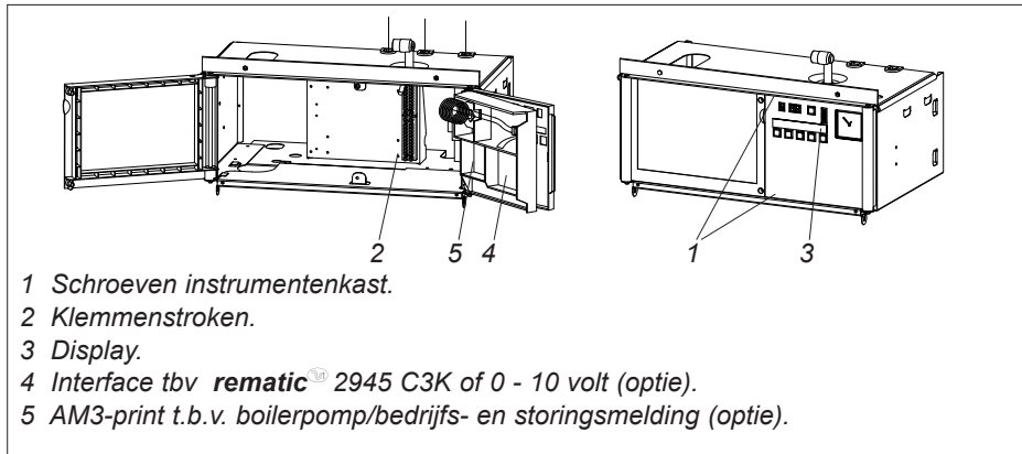
Afb. 19 Gesloten en geopende instrumentenkast 00.V3H.79.00054
