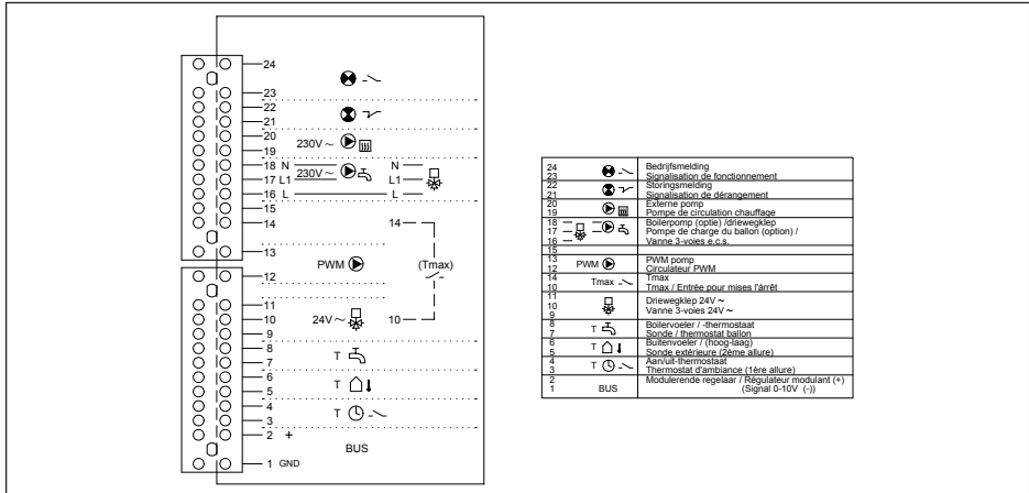
fig. 16 Bornier de raccordement
