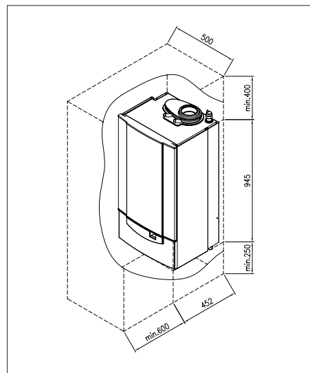
fig. 06 Espace libre pour montage
