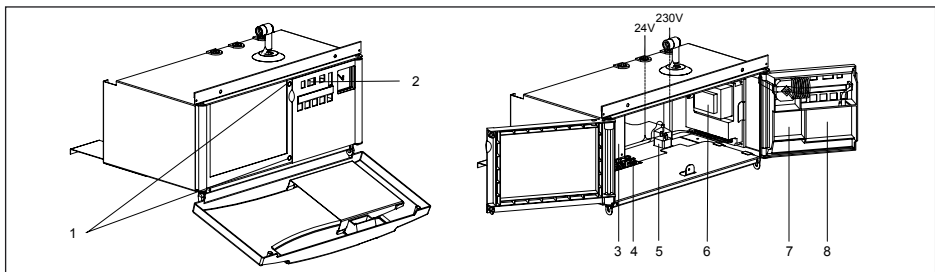
fig. 17 Tableau de bord, vues interne et externe.
