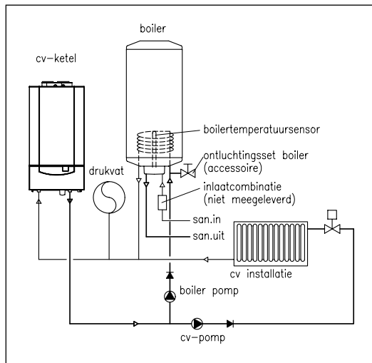
afb. 12 Aansluiting boiler m.b.v. boilerpomp.
