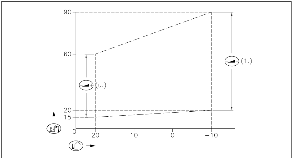
afb. 21 Interne stooklijn
