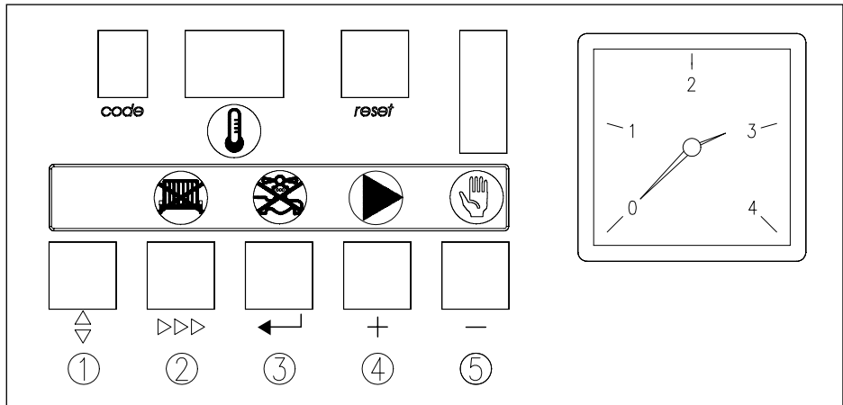
afb. 04 Display 00.W4H.79.00044
