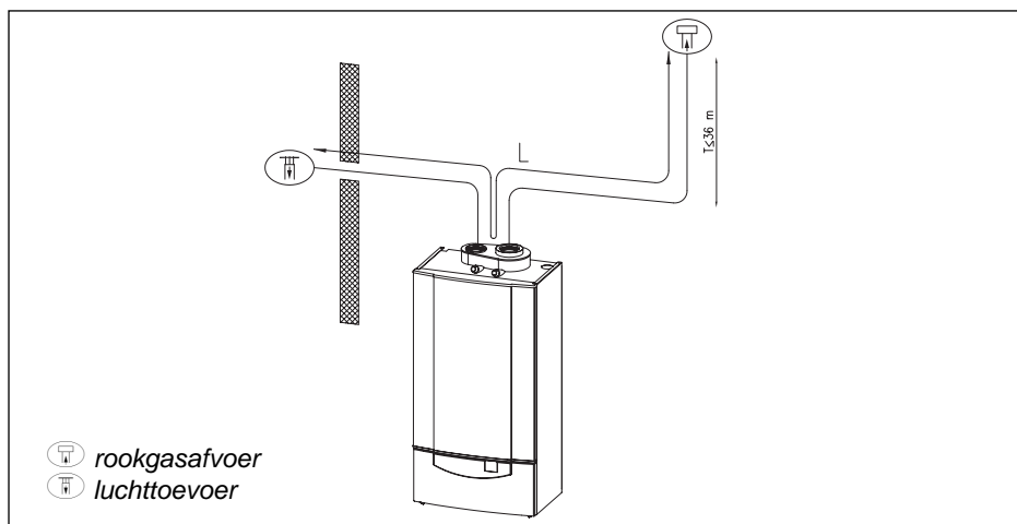
afb. 11 Uitmondung in verschillende drukgebieden.
