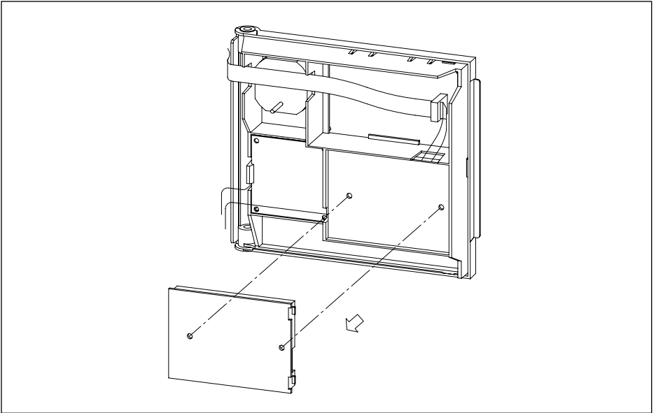
afb. 17 Interface inbouw
