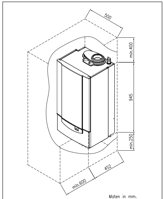
afb. 06 Opstellingsruimte Remeha Quinta 85
