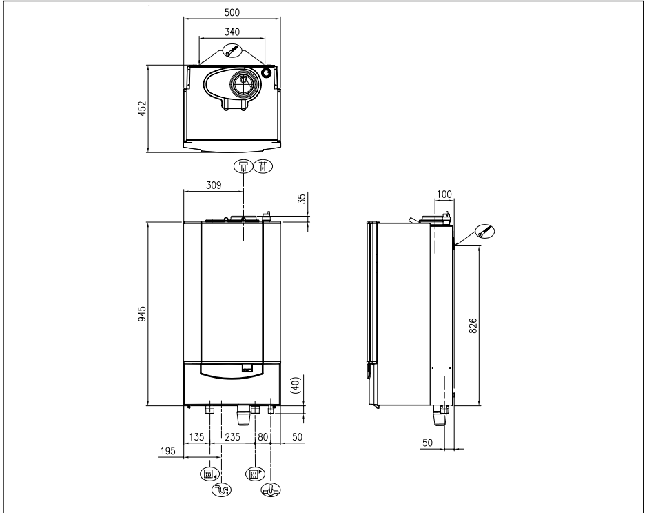
afb. 02 Afmetingen Remeha Quinta 85
