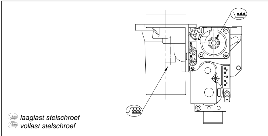
afb. 23 Instelpunten
