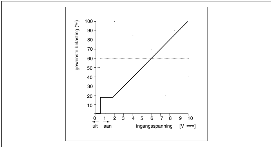
afb. 20 Relatie tussen ingangsspanning en nominale belasting
