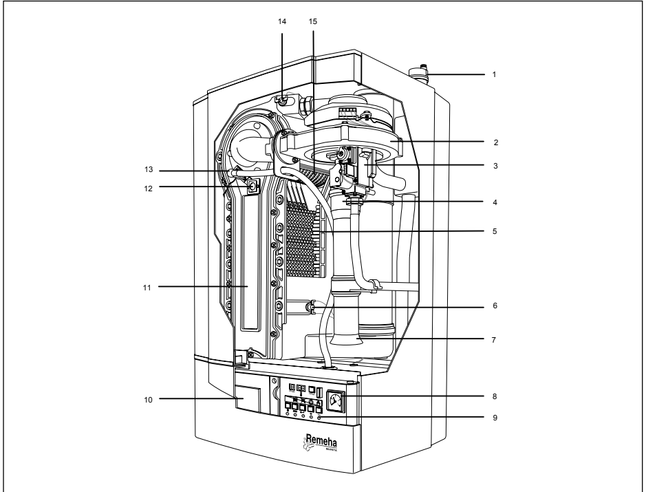
afb. 01 Toesteluitvoering
