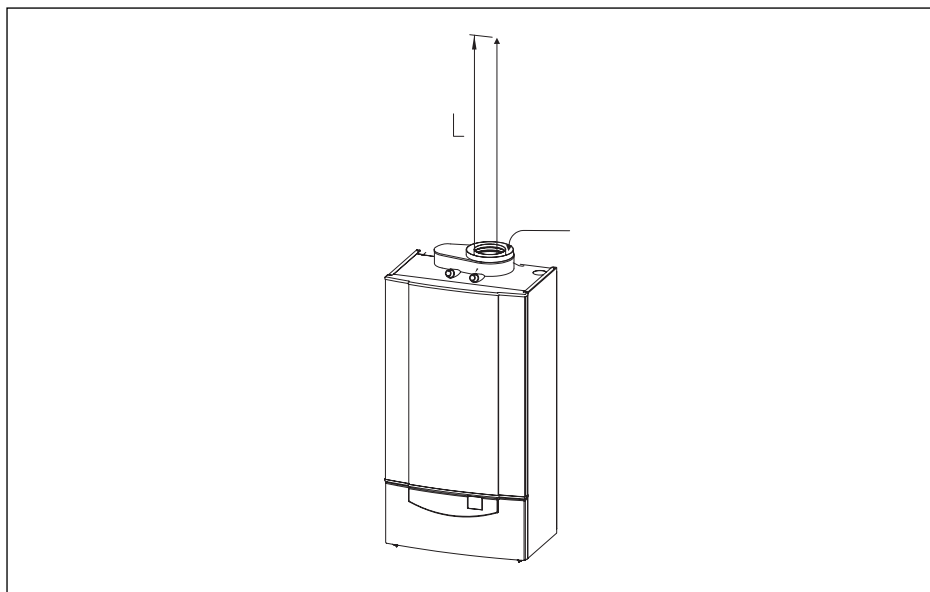
afb. 09 Standaardsituatie 'open uitvoering'
