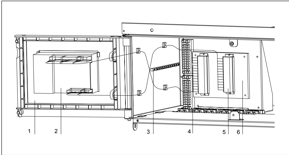
afb. 18 Geopende instrumentenkast met gemonteerde rematic ® 2945 C3K en adapter
