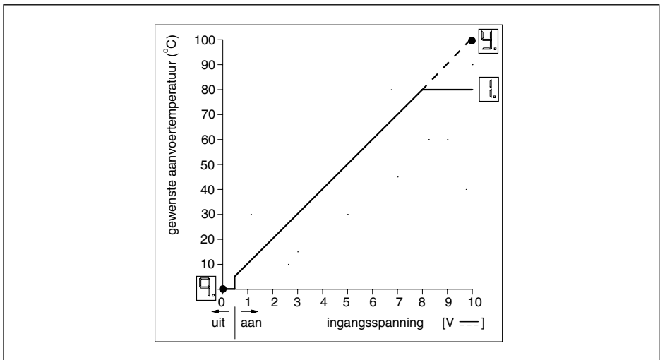
afb. 19 Relatie tussen ingangsspanning en temperatuur
