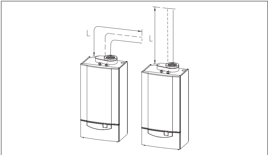
afb. 10 Standaardsituaties 'gesloten uitvoering'
