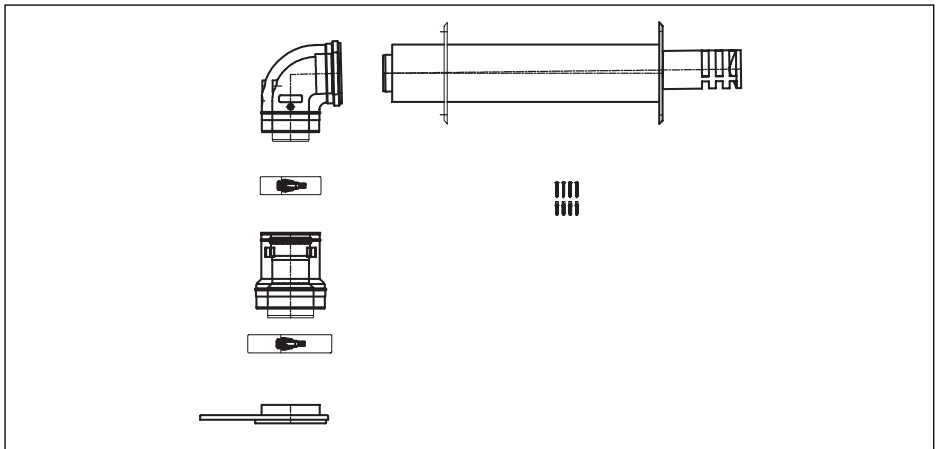
afb. 08 Remeha geveldoorvoerset
