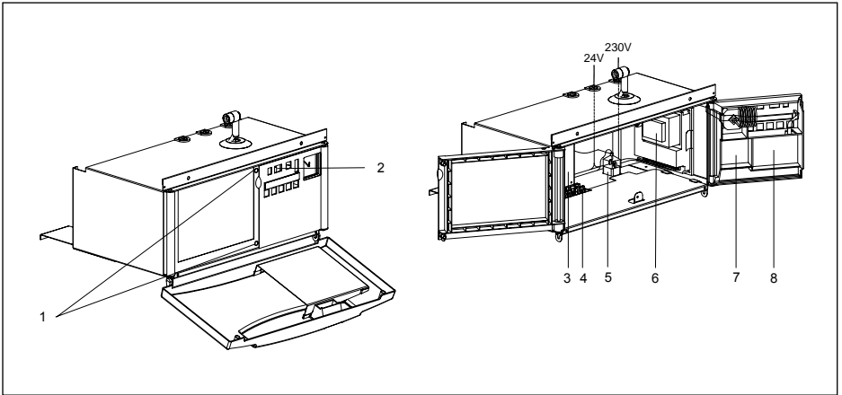
afb. 16 Gesloten en geopende instrumentenkast
