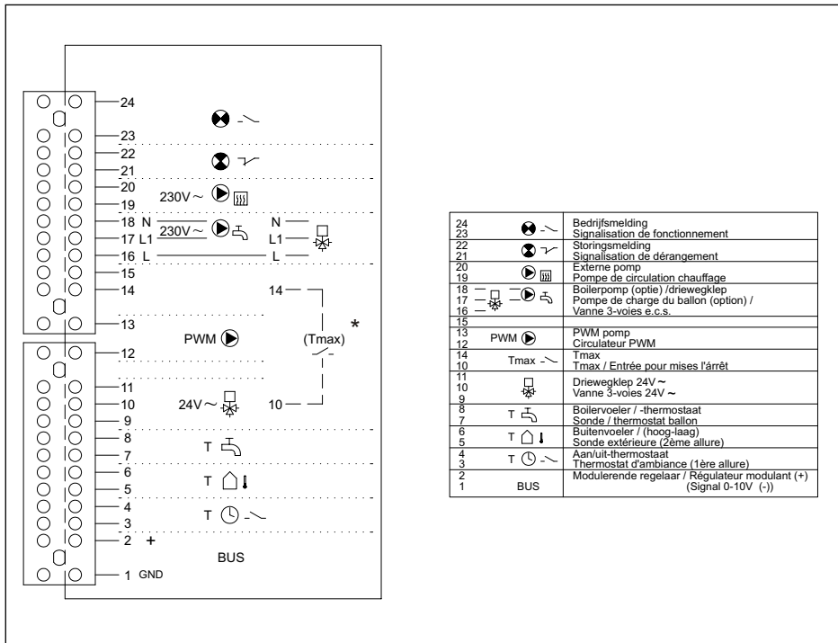
afb. 15 Klemmenstrook
