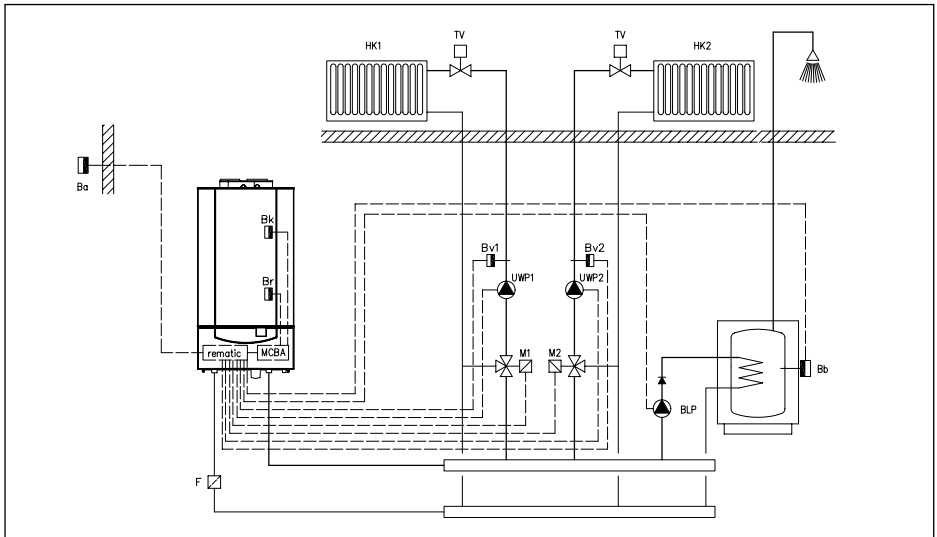
afb. 13 Gesloten verdeler met rematic ® -regelaar.
