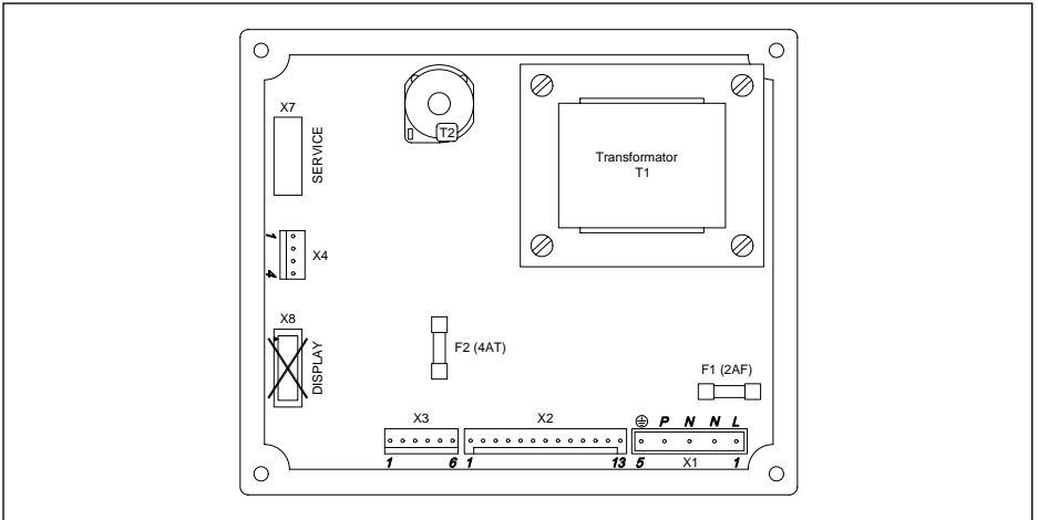
afb. 14 Beveiligingsautomaat Gasmodul met reservezekeringen
