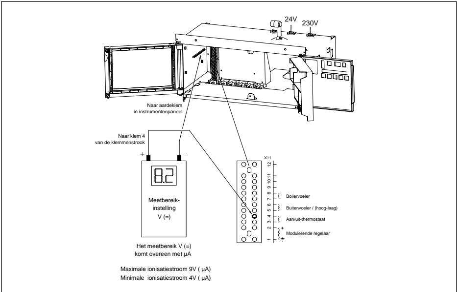
afb. 25 Ionisatiemeting
