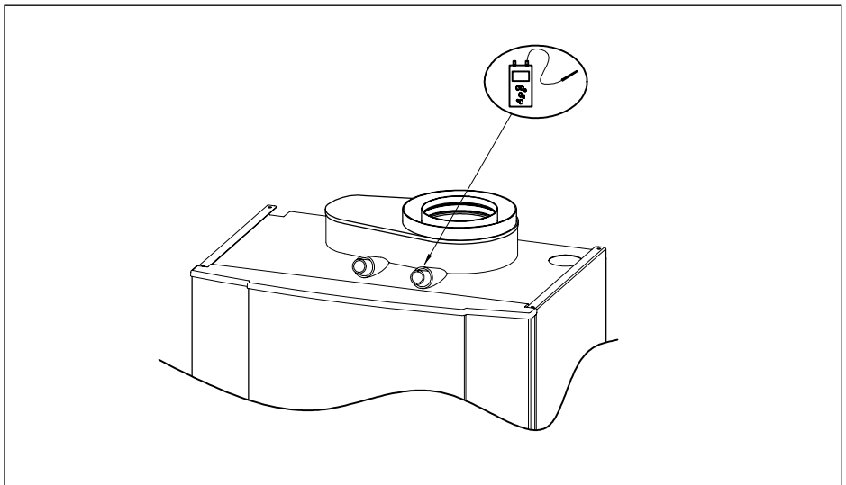
afb. 24 Rookgasmeetpunt
