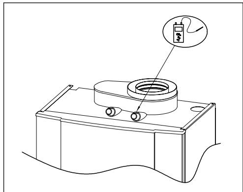
afb. 22 Rookgasmeetpunt
