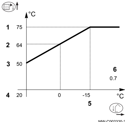
Abb. Heizkennlinie 101
