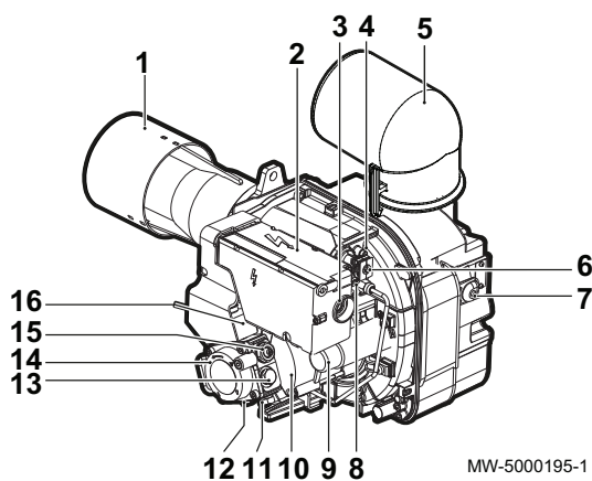
Abb.11 Hauptkomponenten
