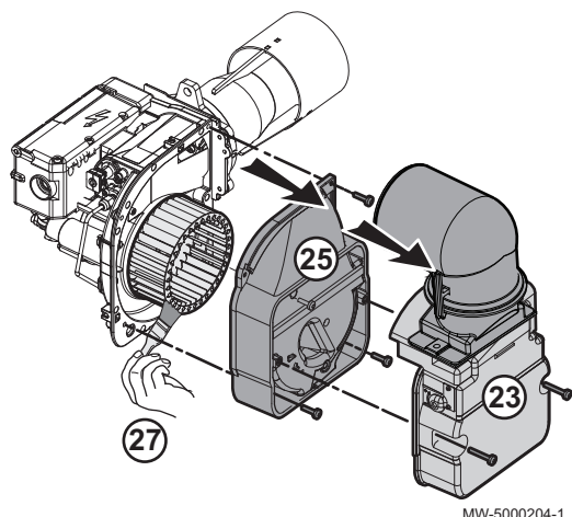
Abb. 121 Reinigung des Gebläses
