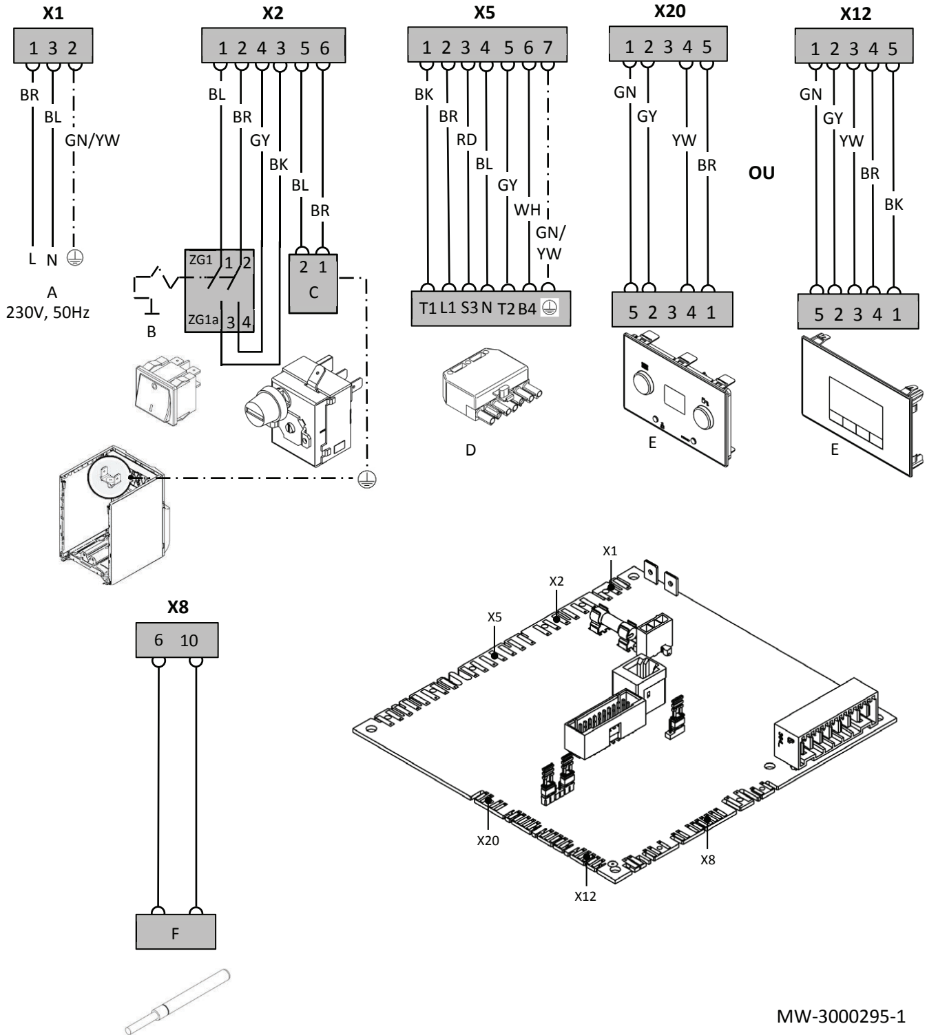
Abb.4 Elektrischer Schaltplan
