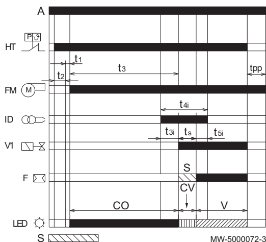
Abb.6 Normaler Betrieb
