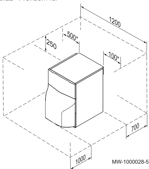
Abb.22 Freiraum für
