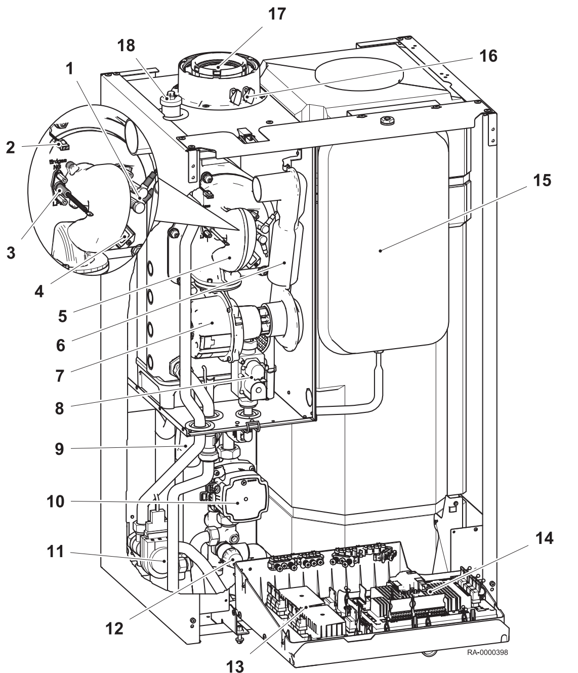
Fig.3 Vue de la chaudière WGB-K EVO (représentée sans la paroi avant et le couvercle du régulateur)
