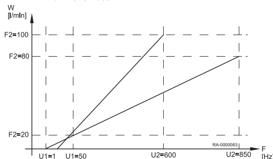
Fig.30 Exemple de deux courbes de capteur différentes
