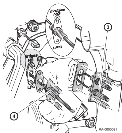
Fig.34 Retrait de l'électrode d'allumage et d'ionisation
