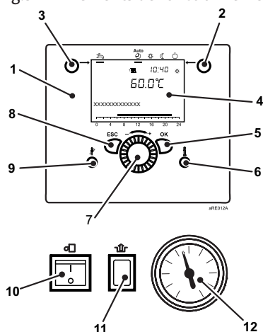
Fig.5 Éléments de fonctionnement
