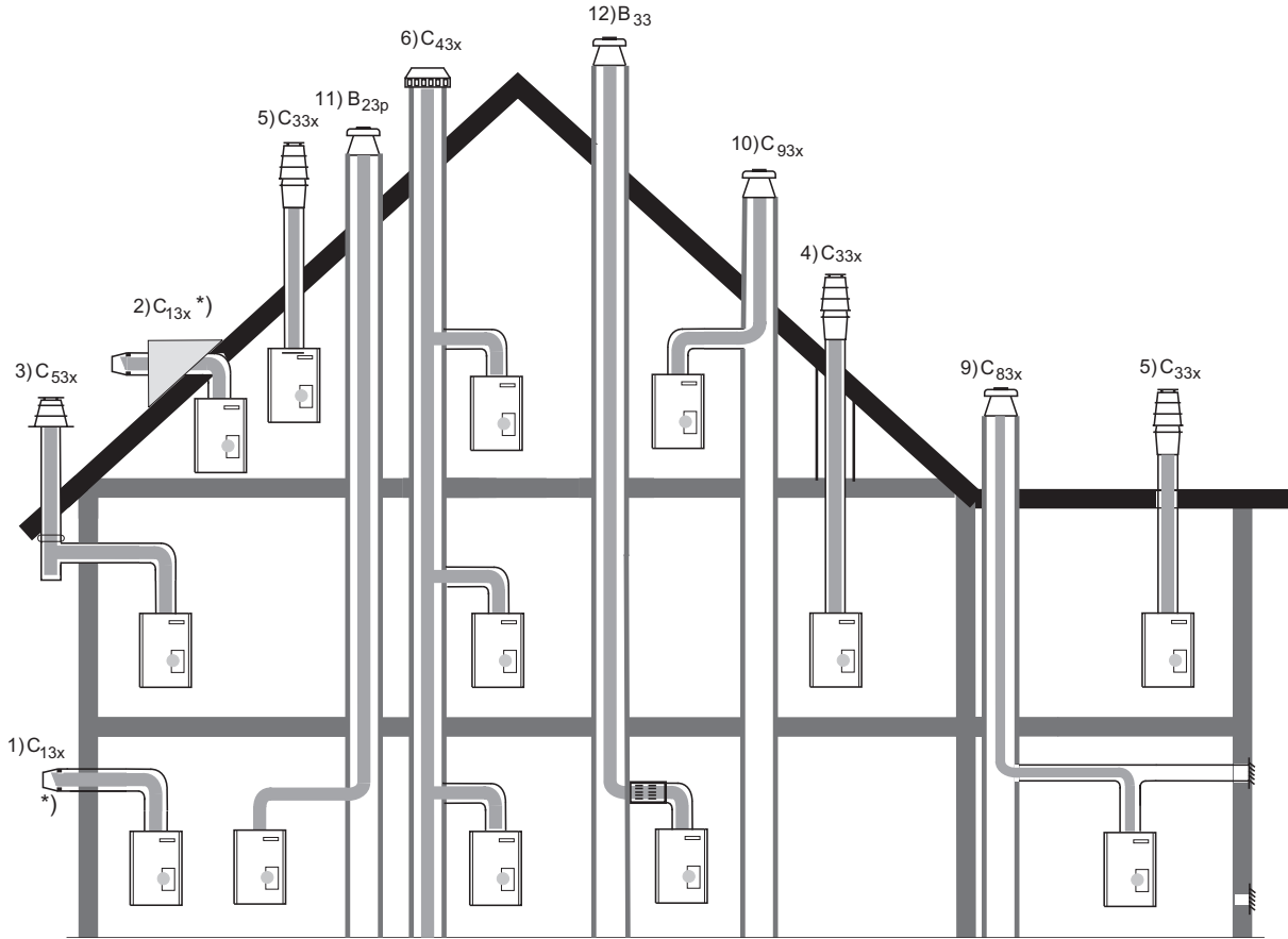
Fig.13 Possibilités de raccordement avec KAS (accessoire)
