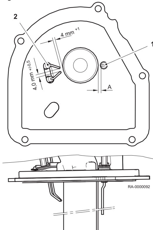
Fig.33 Électrodes
