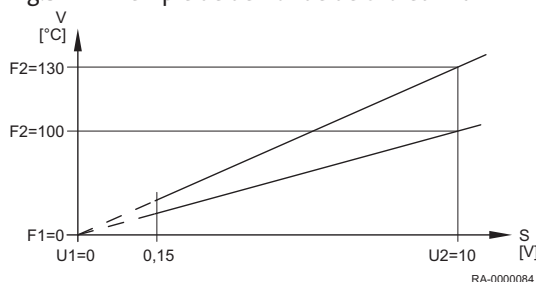
Fig.31 Exemple de demande de chaleur 10 V
