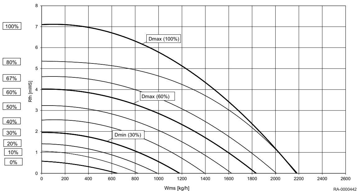
Fig.1 Hauteur manométrique disponible WGB-K EVO pour le circuit de chauffage de pompage
