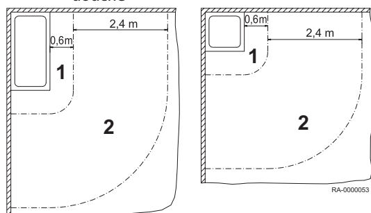
Fig.8 Espaces dans les salles de bains et de douche
