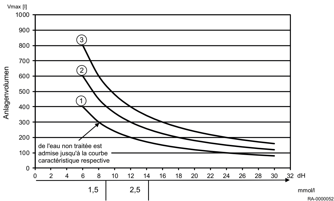
Fig.7 Diagramme de dureté de l'eau
