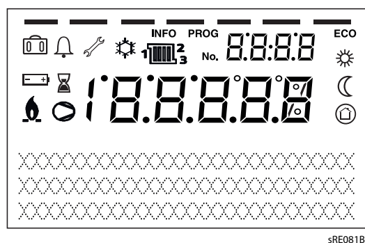
Fig.6 Symboles sur l'afficheur
