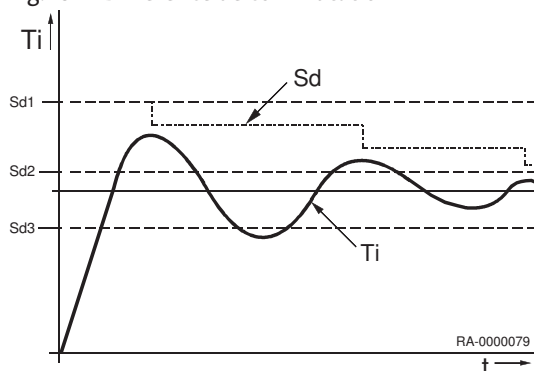
Fig.28 Différence de commutation
