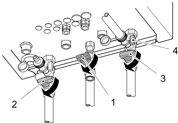
Afb. 6: Afsluitkleppen en gasafsluitkraan sluiten
