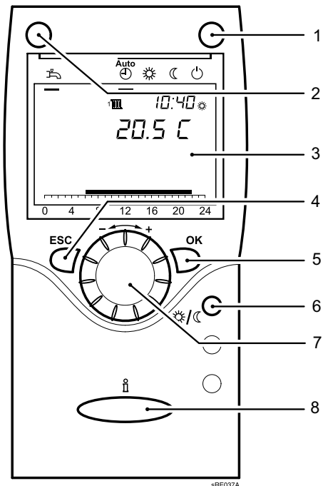
Fig 35: Interface utilisateur des appareils ambiants RGT
