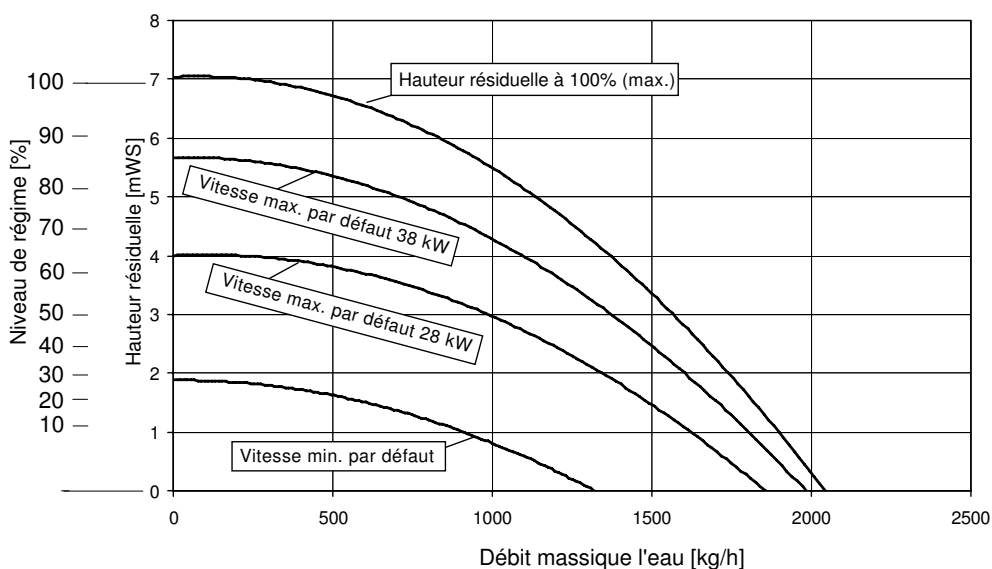
Fig 26: Hauteur manométrique résiduelle WGB 28/38 E
