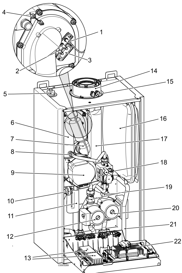
Fig 37: Vue de la chaudière WGB (représentation sans panneau avant et recouvrement de la régulation)
