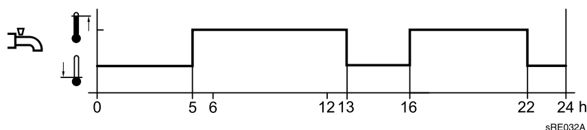
Fig 28: Libération selon le programme de commutation de temps 4 (exemple)
