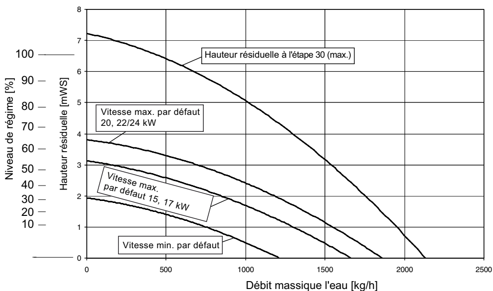
Fig 25: Hauteur manométrique résiduelle WGB 15/20 E
