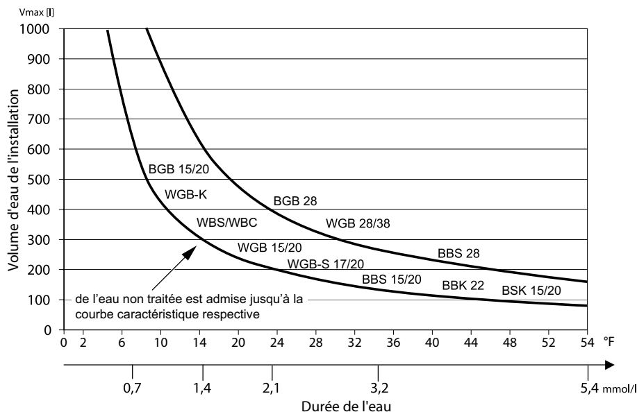
Fig 2: Diagramme hydrotimétrique
