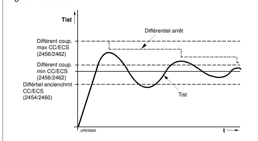
Fig 29: Différentiel
