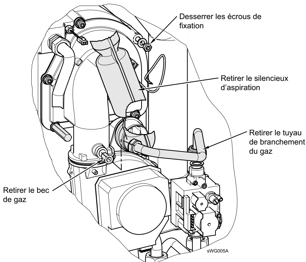
Fig 36: Démontage du brûleur à gaz
