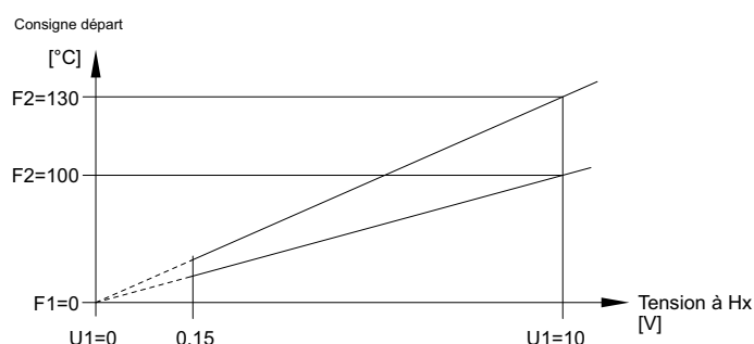
Fig 34: Exemple pour la demande de chaleur 10 V et la demande de froid 10 V
