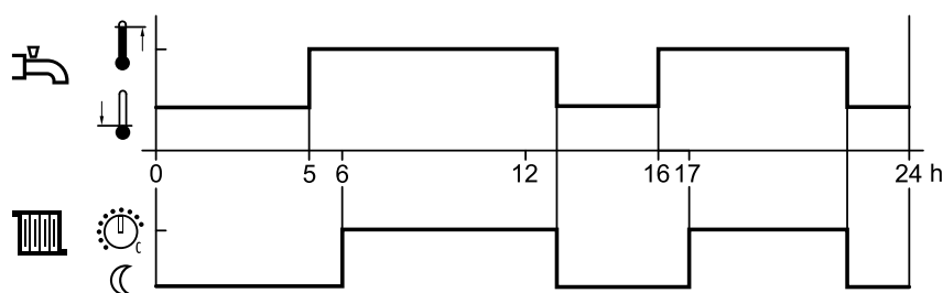
Fig 27: Libération en fonction des programmes de commutation de temps des circuits de chauffe (exemple)
