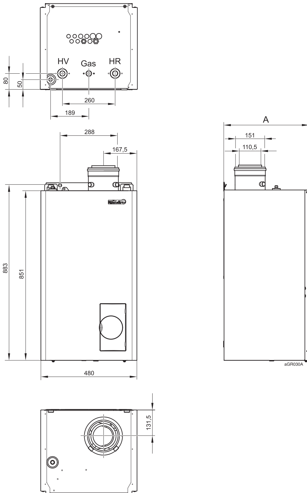
Schets 1: afmetingen en aansluitingen
