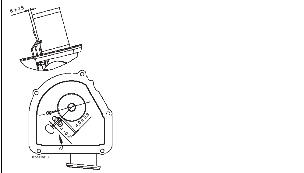
Schets 23: elektroden
