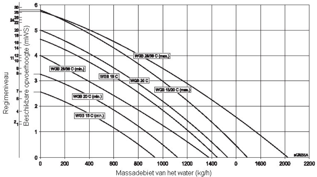
Schets 14: beschikbare manometrische opvoerhoogte
