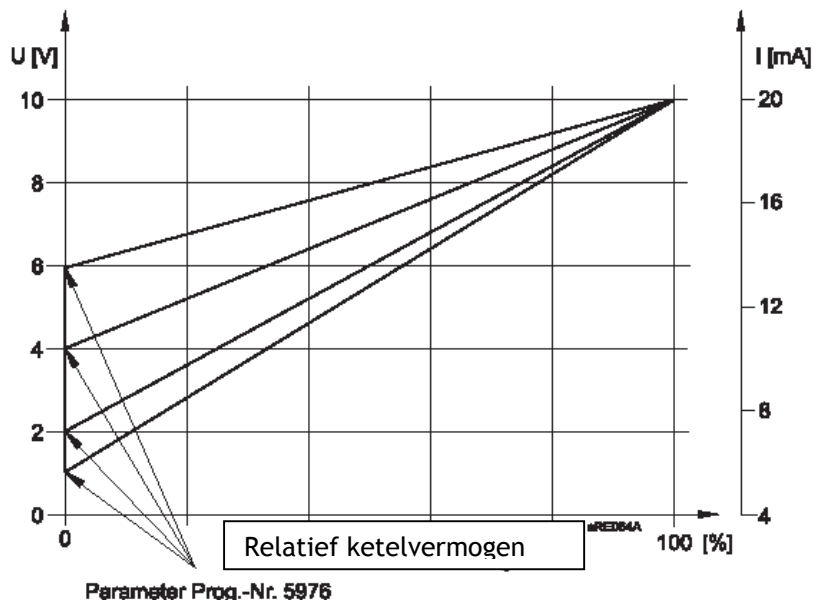
Schets 18: vermogensinstelling
