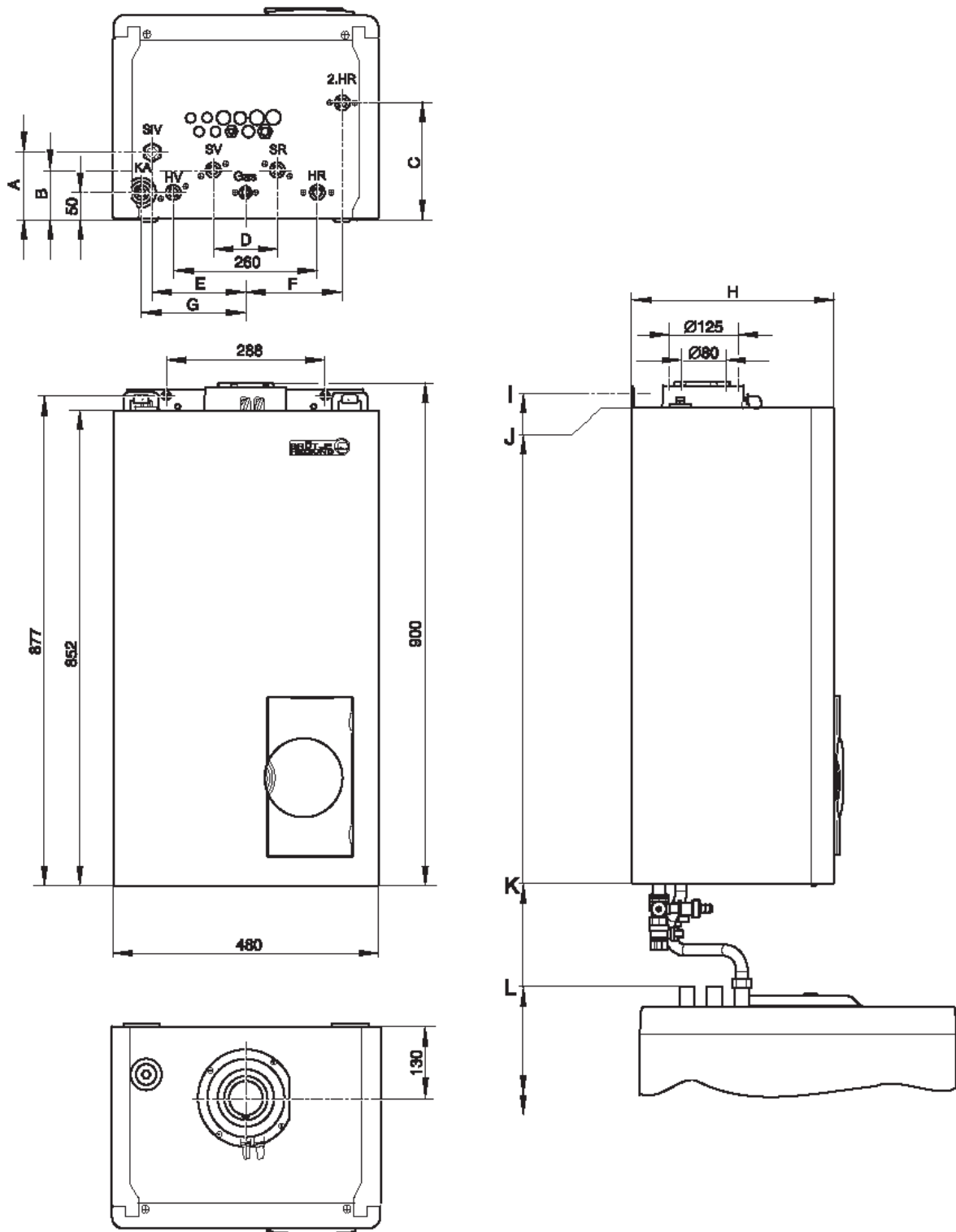
Schets 1: afmetingen en aansluitingen
