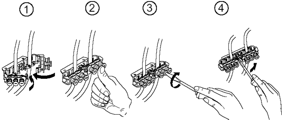
Schets 9: kabelhalzen
