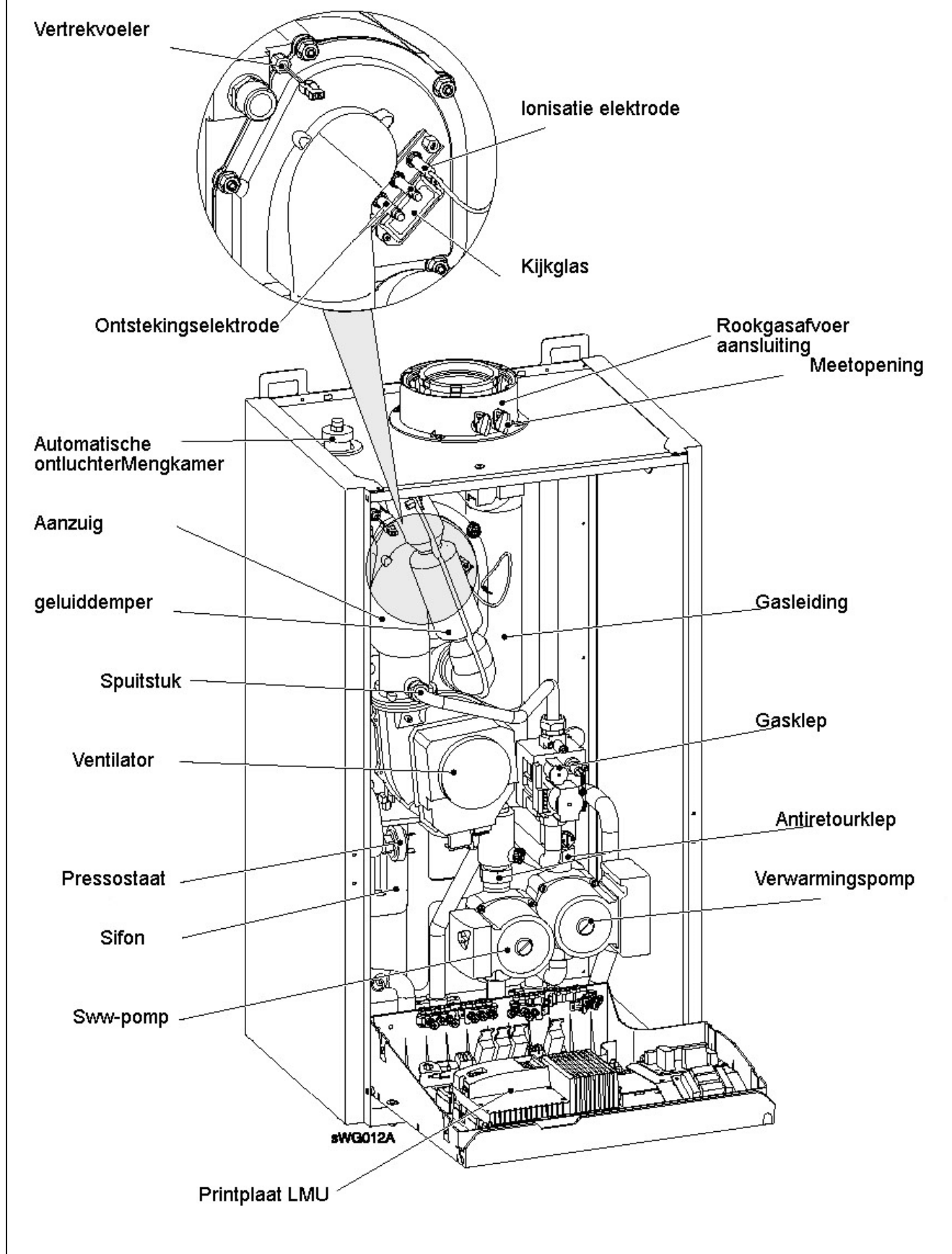
Schets 22: doorzicht van de ketel WGB 28 / 38 C
