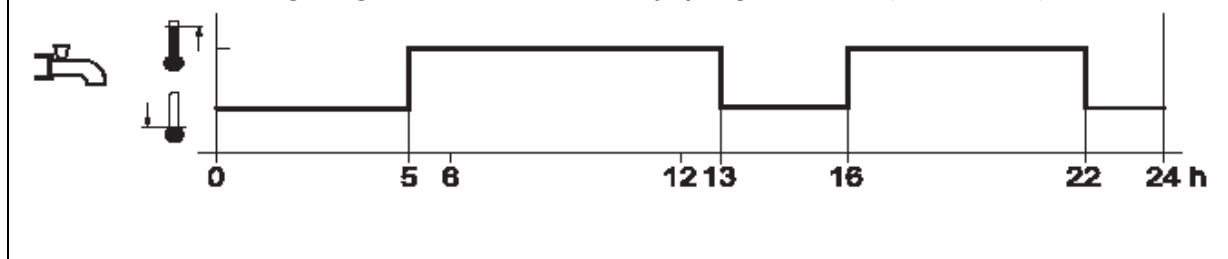
Schets 16: toelating volgens het omschakeltijdprogramma 4 (voorbeeld)
