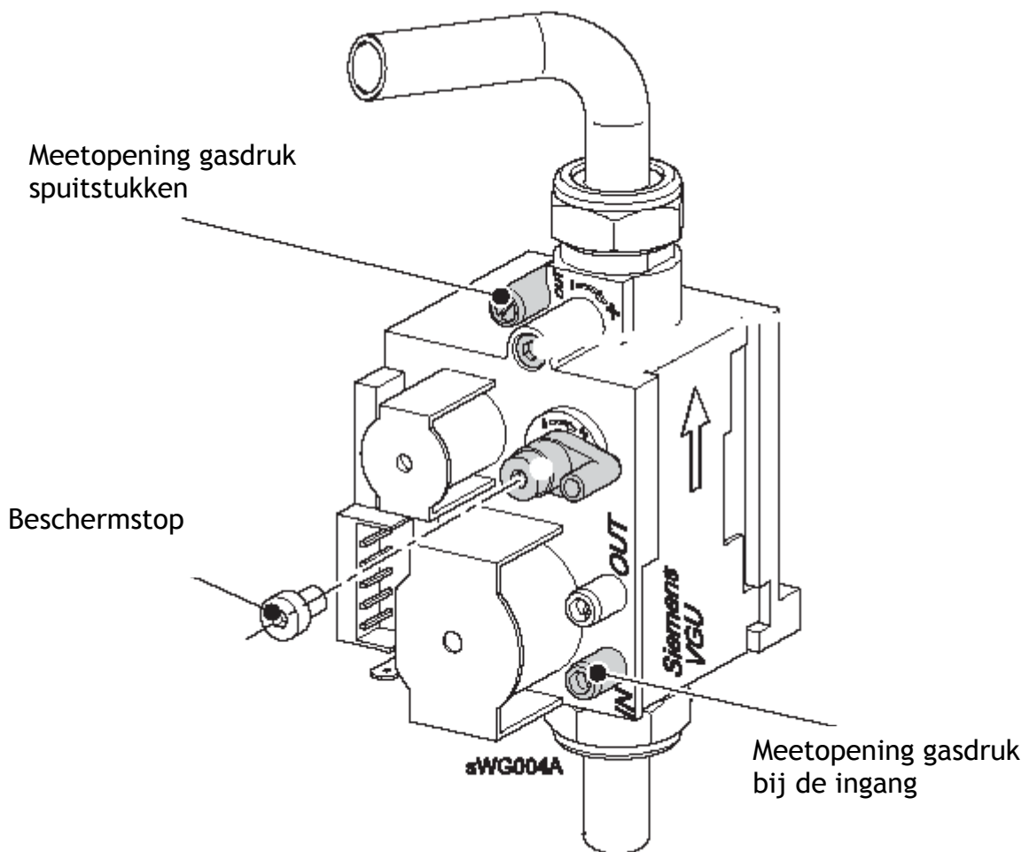
Schets 8: Gasklep
