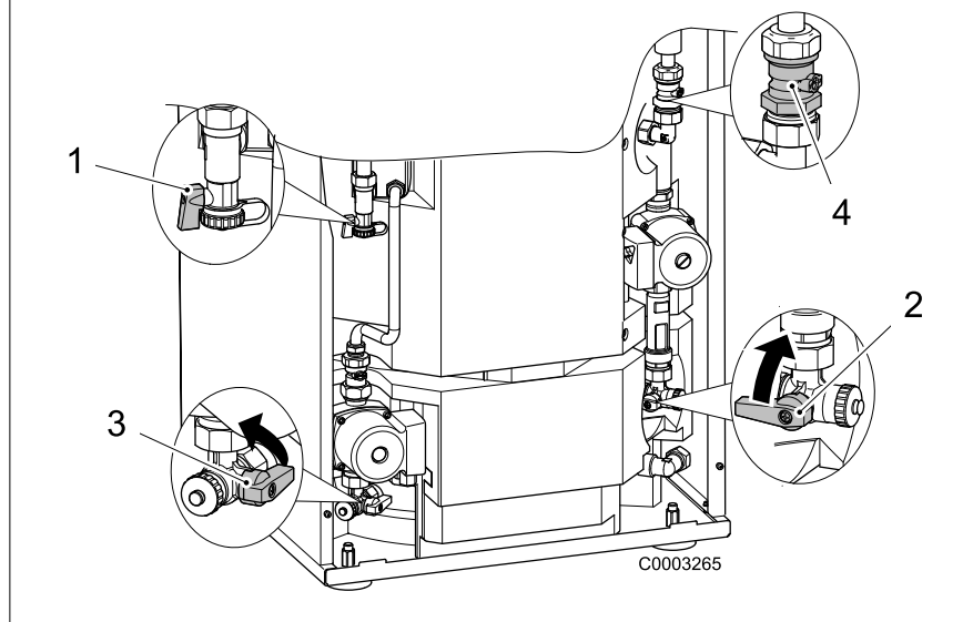
Afb. 7: Verwarming - en tapwater en zonnevloeistof aflaten
