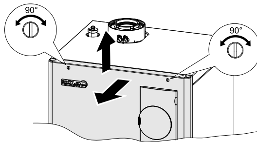
5. Afb. 6: Demontage van de ketelmantel
