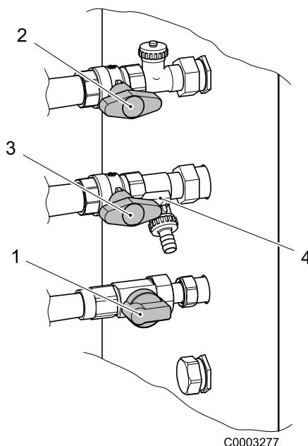
Afb. 5: Afsluitkleppen en gasafsluitkraan sluiten
