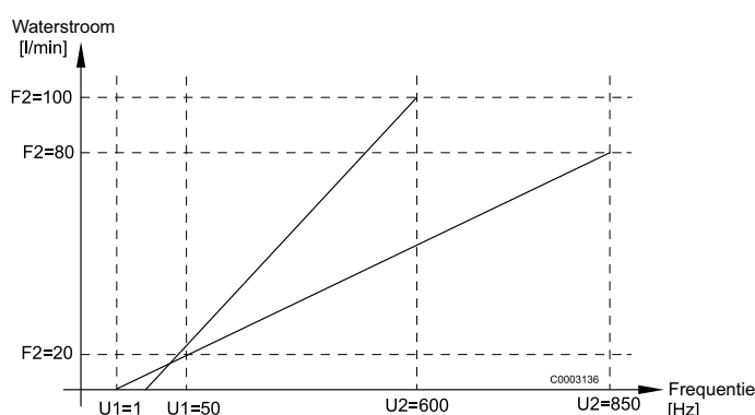
Afb. 29: Voorbeeld voor twee verschillende voelerswaarden
