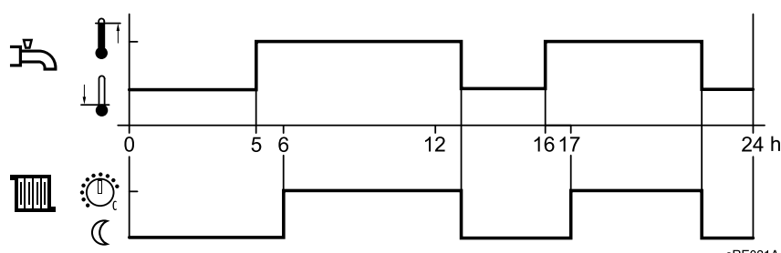
Afb. 23: Vrijgave steeds naargelang de tijdschakelprogramma's van de verwarmingscircuits (voorbeeld)
