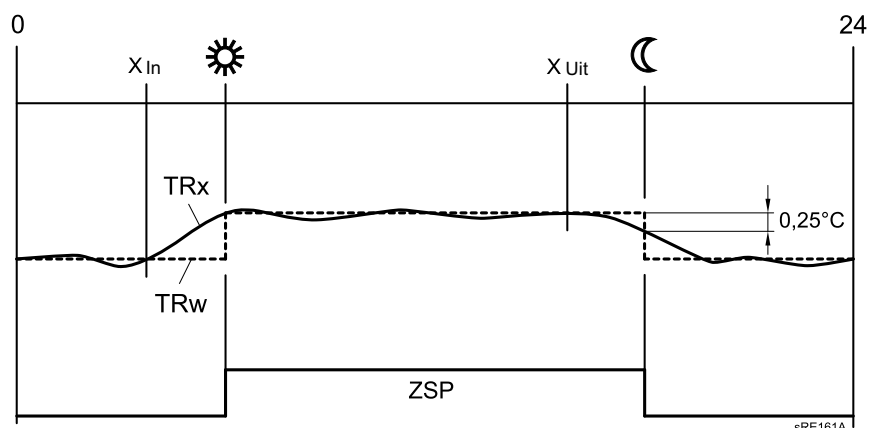
Afb. 19: Inschakel- en uitschakeloptimalisering
