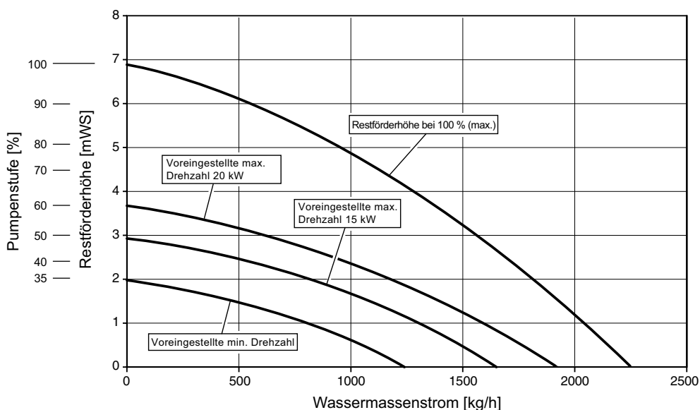
Afb. 22: Beschikbare opvoerhoogte BGB 15-28 E
