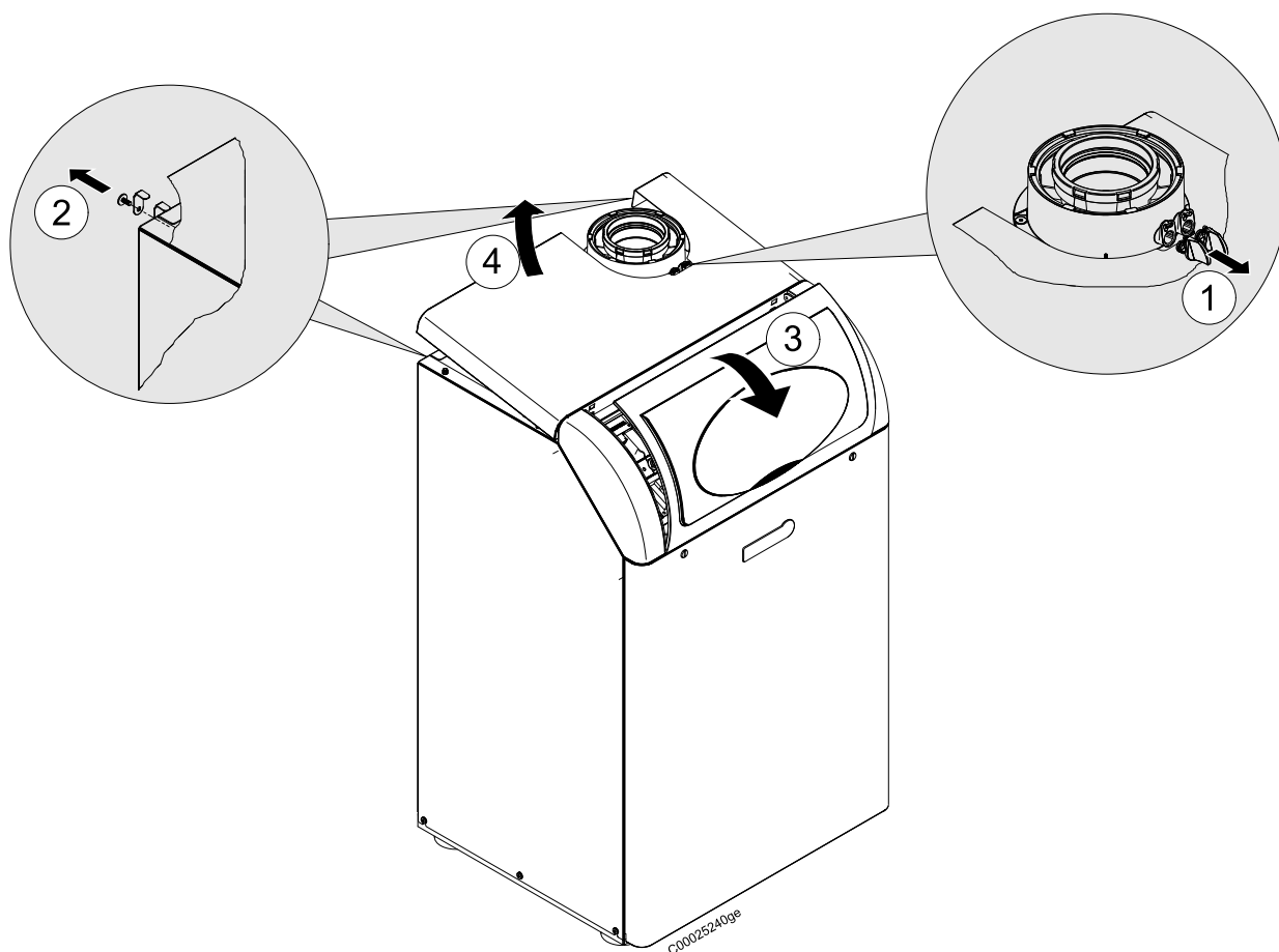
Afb. 33: Beplating als aangegeven demonteren
