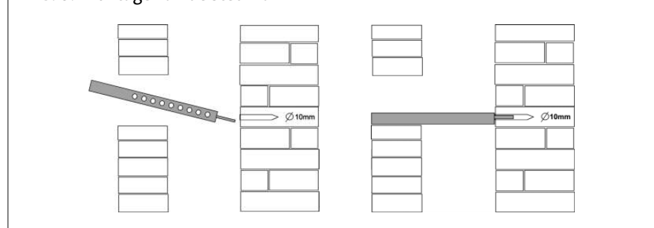
Afb. 8: Montage van de steunrail
