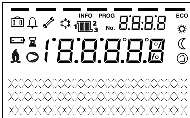
Afb. 14: Symbolen in het display
