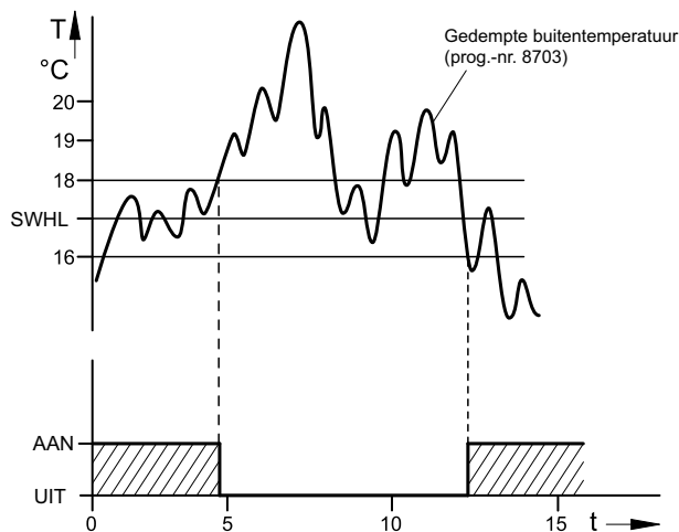
Afb. 16: Zomer/Winter verw grens
