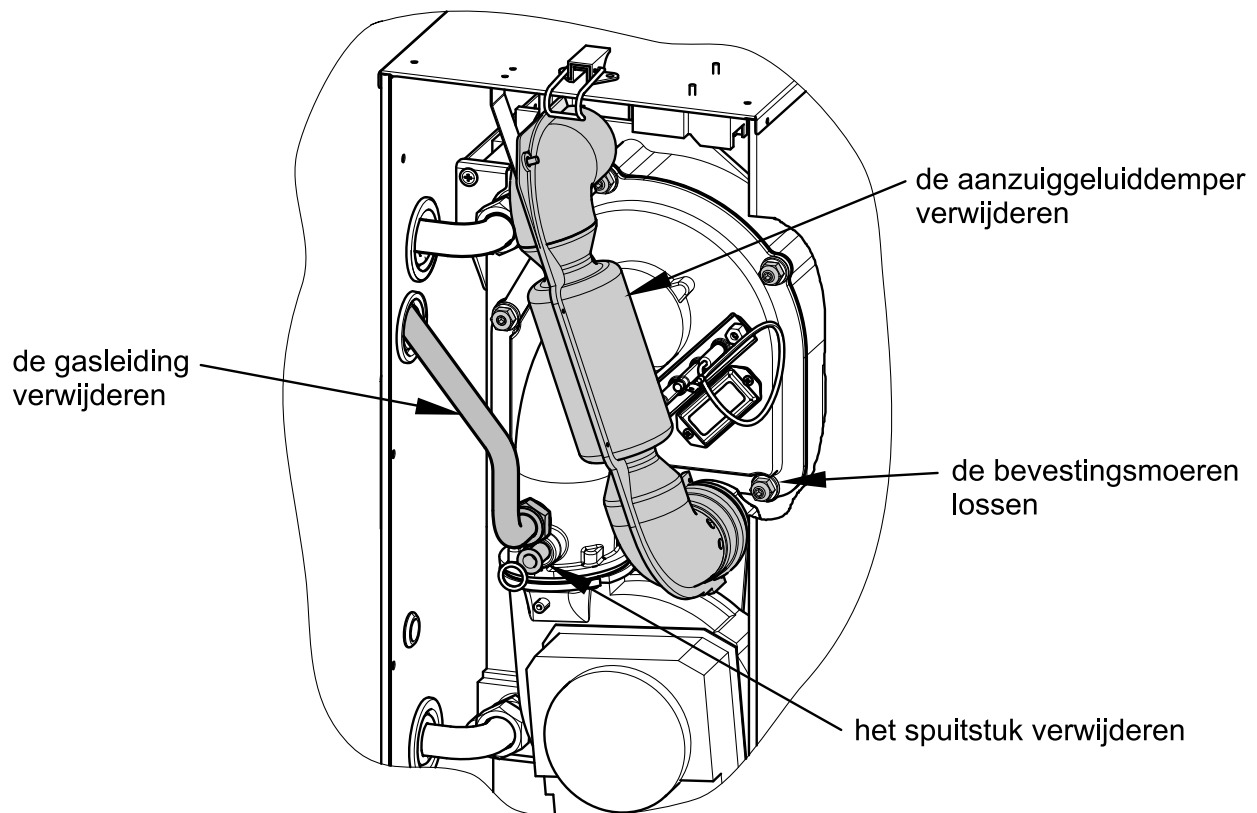
Afb. 32: Demontage van de gasbrander
