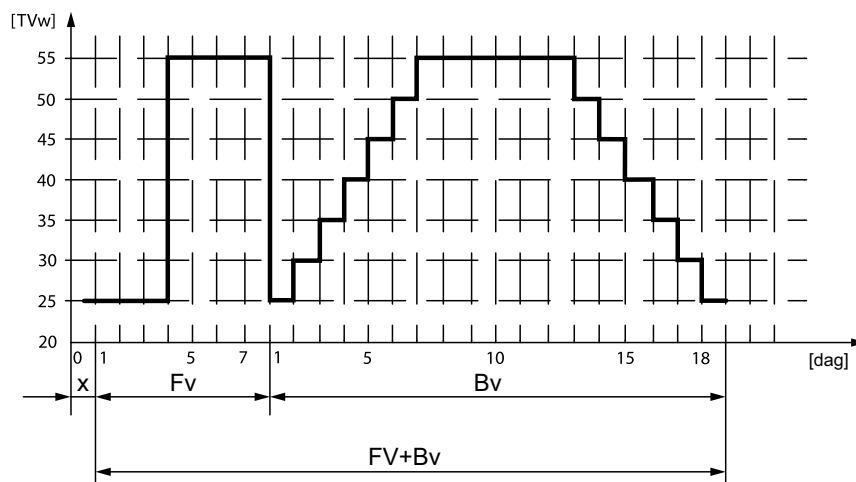
Afb. 21: Temperatuurprofiel bij de estrik-drogingsfunctie
