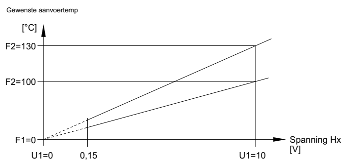
Afb. 30: Voorbeeld bij warmtevraag 10 V en koude vraag 10 V
