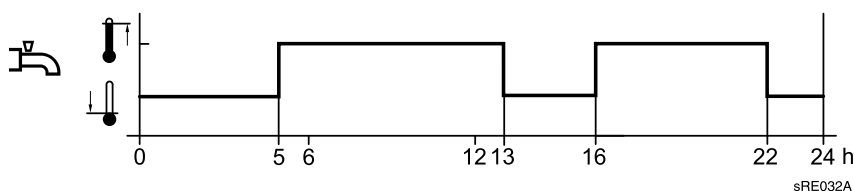
Fig 24: Libération selon le programme de commutation de temps 4 (exemple)
