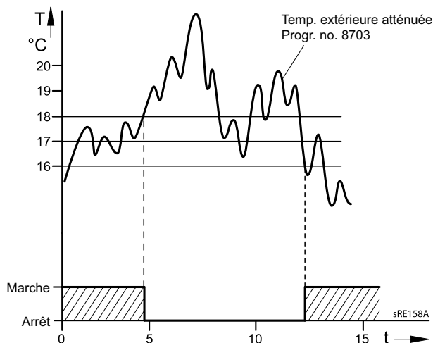
Fig 16: Limite de chauffe été/hiver
