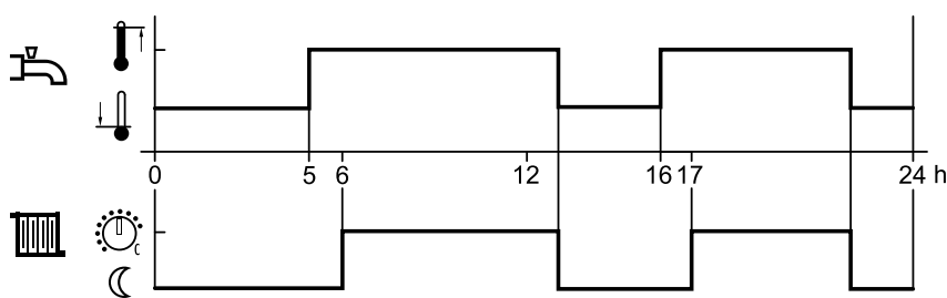
Fig 23: Libération en fonction des programmes de commutation de temps des circuits de chauffe (exemple)
