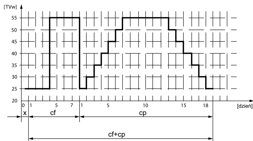
Fig 21: Courbe de température lors de la fonction dessèchement de chape
