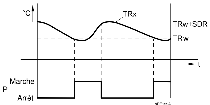
Fig 17: Limit. influence ambiante
