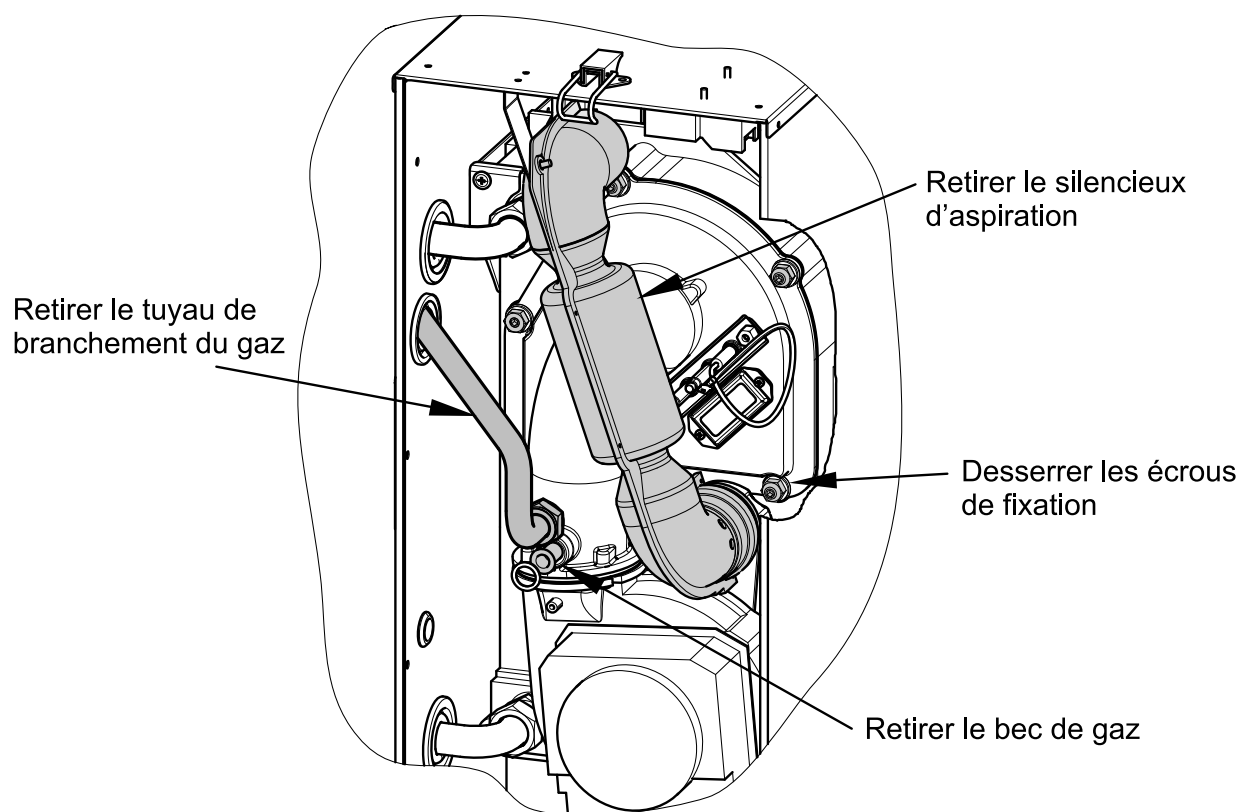
Fig 32: Démontage du brûleur à gaz
