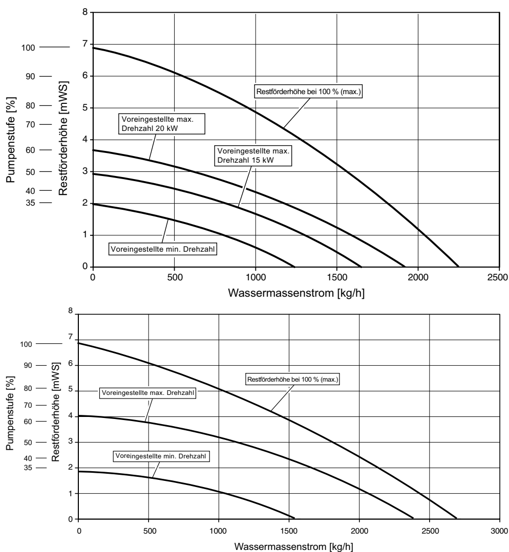
Fig 22: Hauteur manométrique résiduelle BGB 15-28 E
