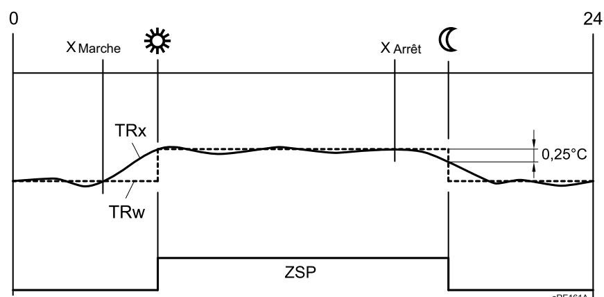
Fig 19: Optimisation à l'enclenchement et optimisation à la coupure
