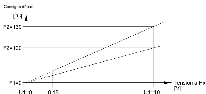
Fig 30: Exemple pour la demande de chaleur 10 V et la demande de froid 10 V
